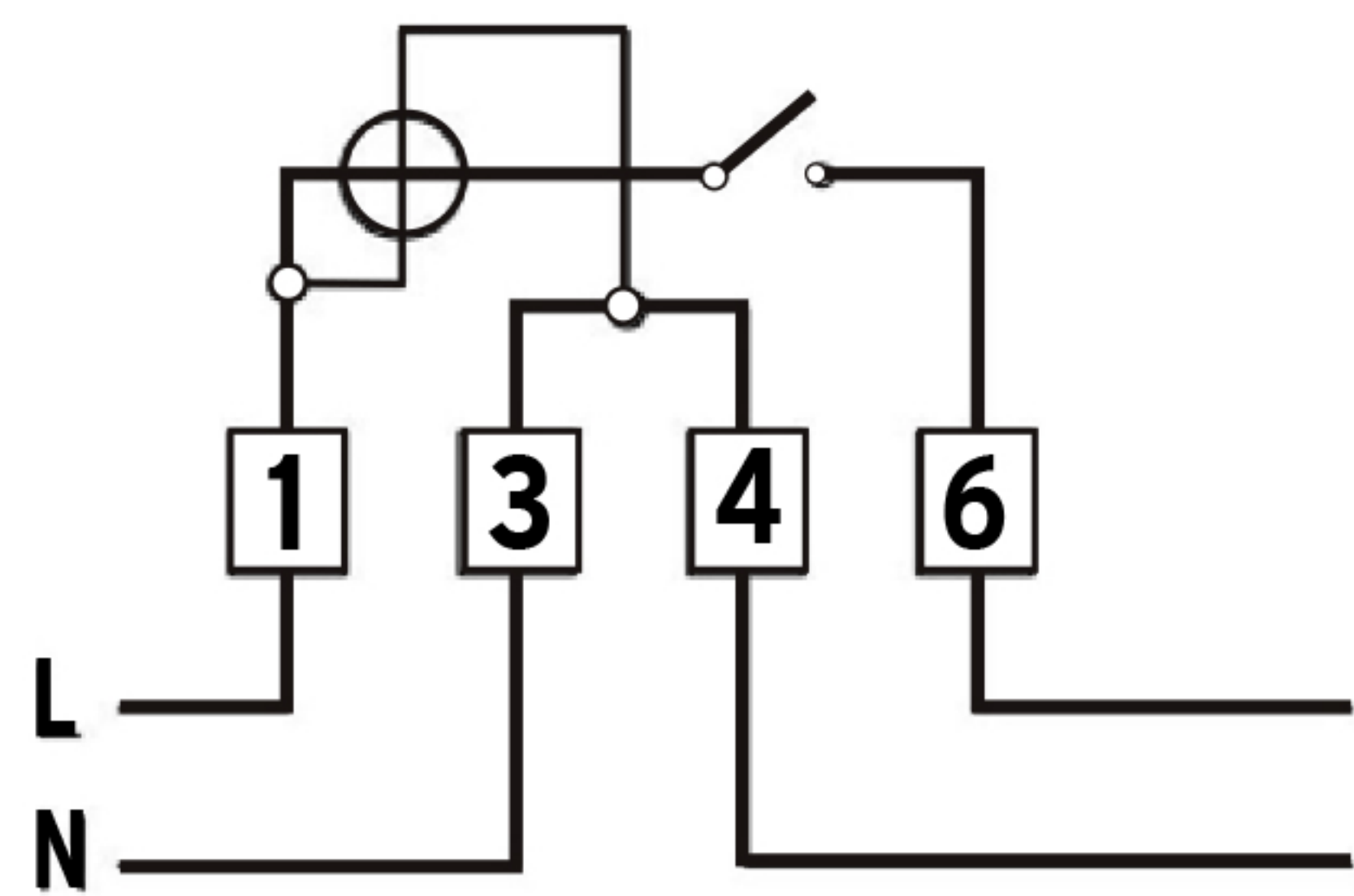
DIAGRAMA DE CONEXIÓN
